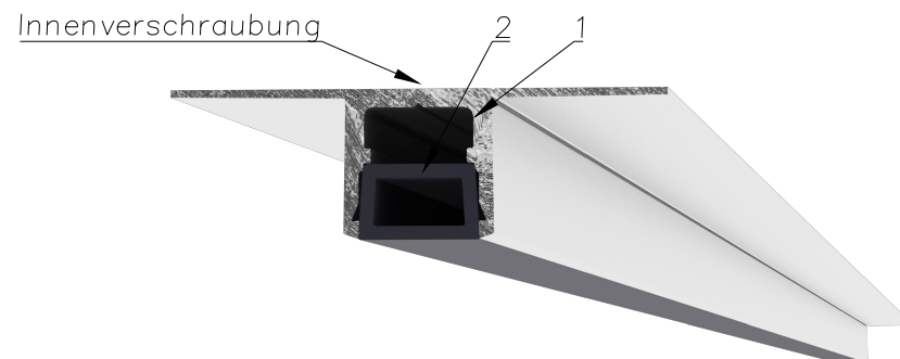
PERSPEKTIVE
